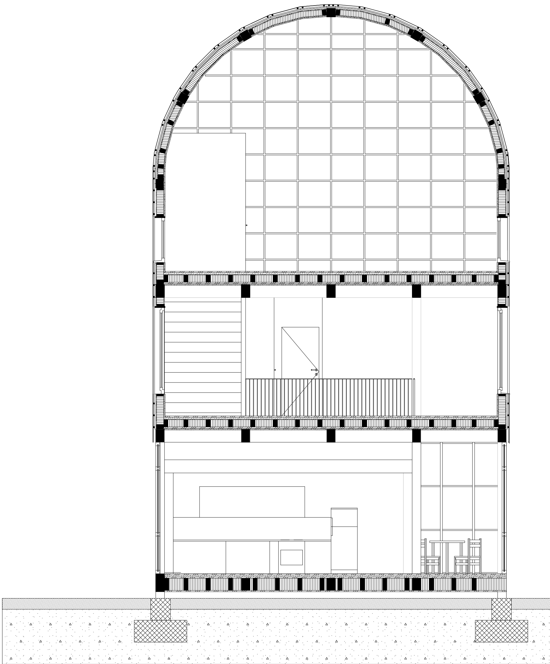
Schnitt S/02
