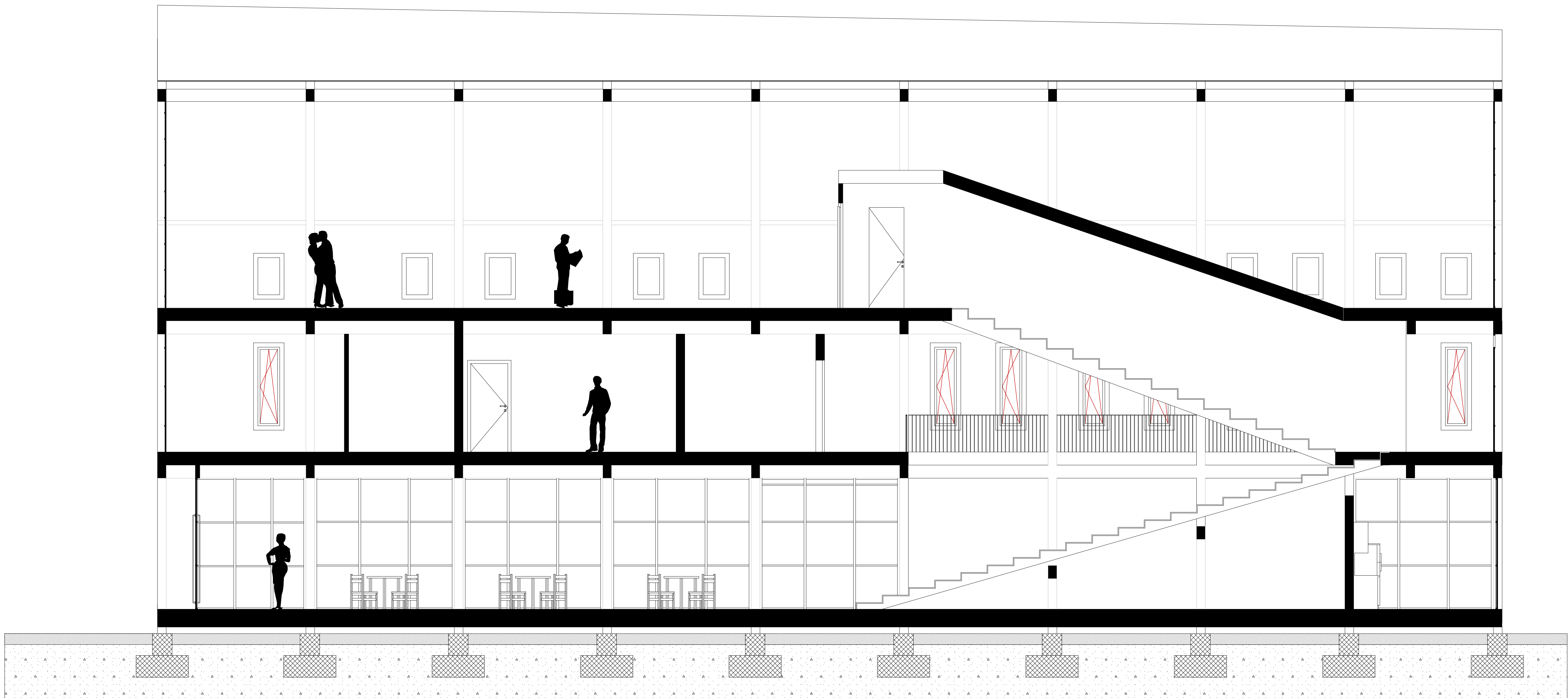
Schnitt S/03
