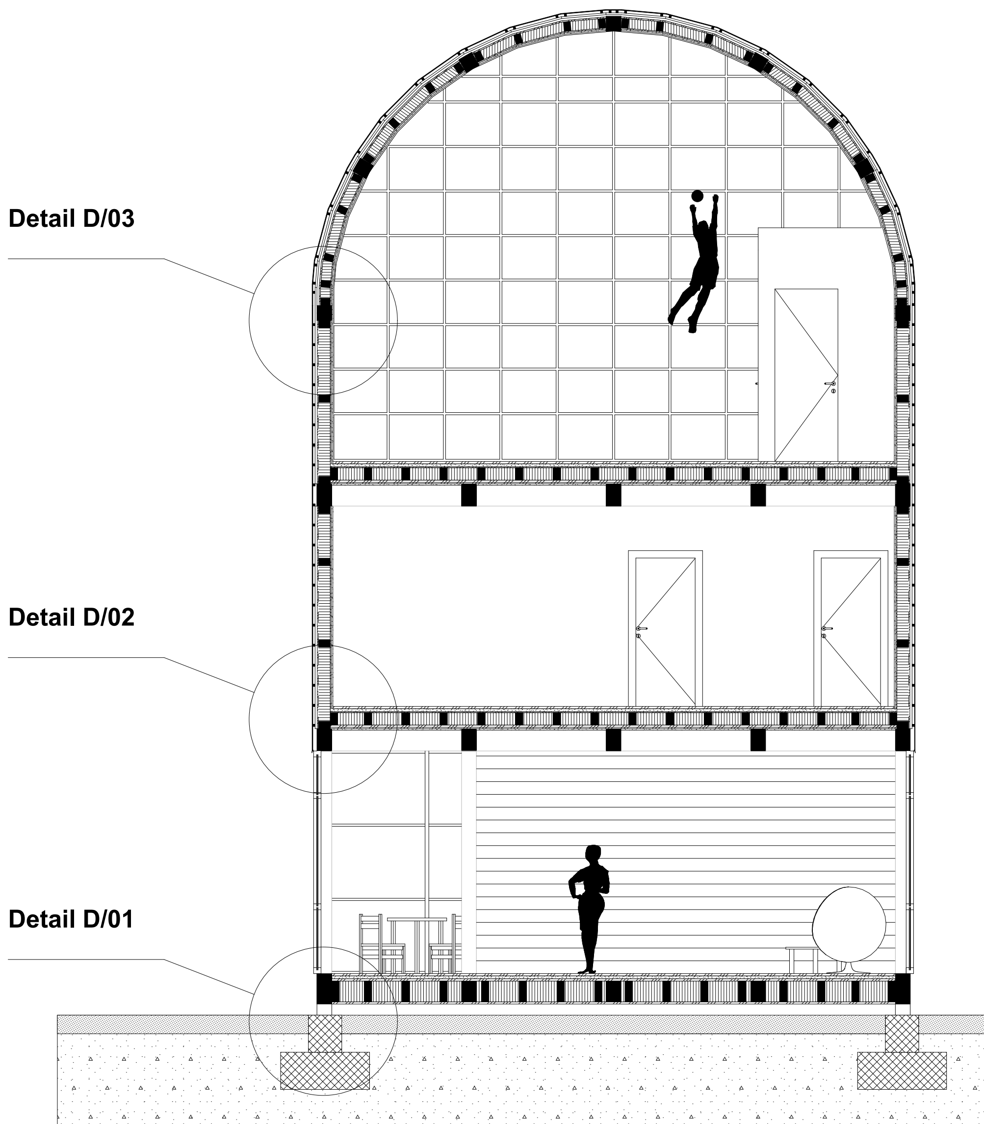
Schnitt S/01
