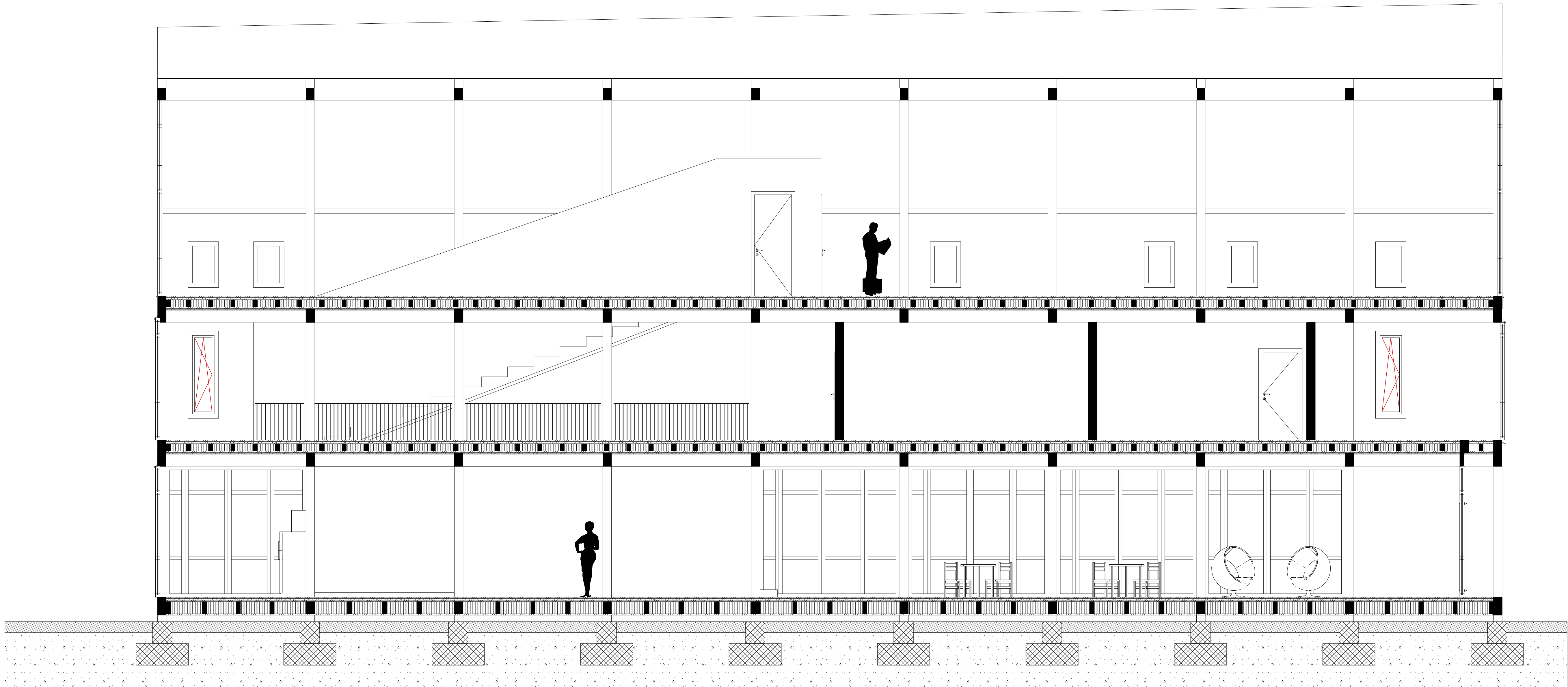
Schnitt S/03
