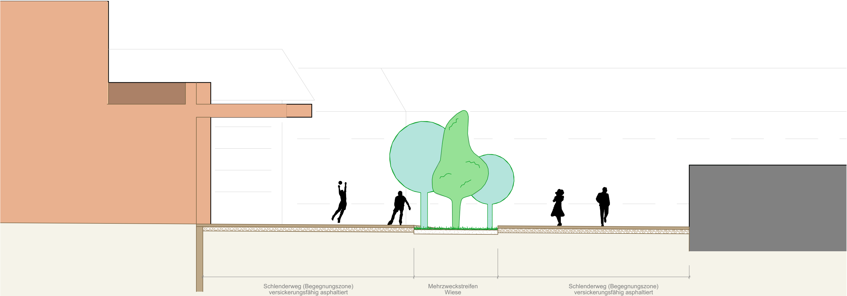
Querschnitt Coop Mst. 1:100
