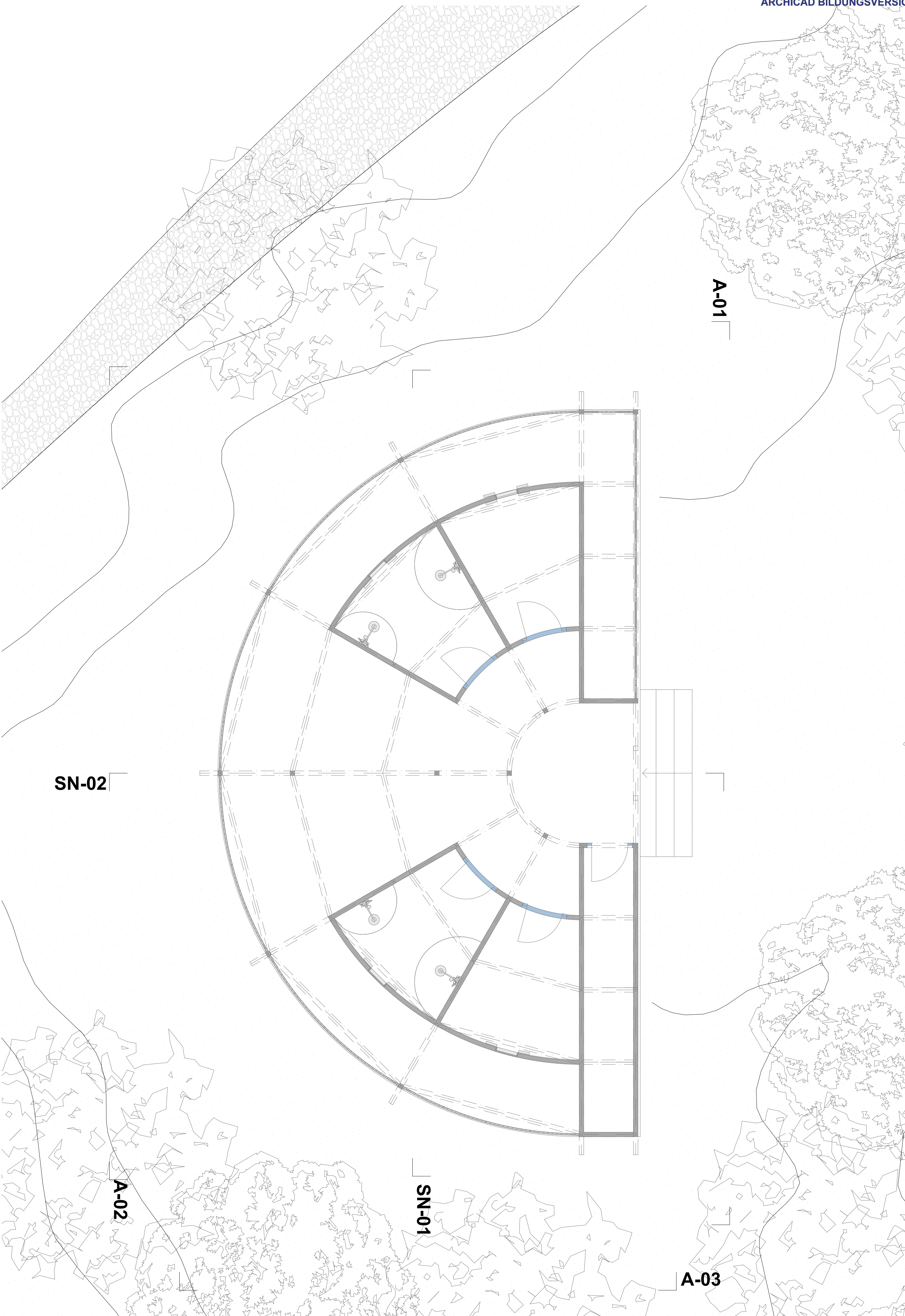
Erdgeschoss
