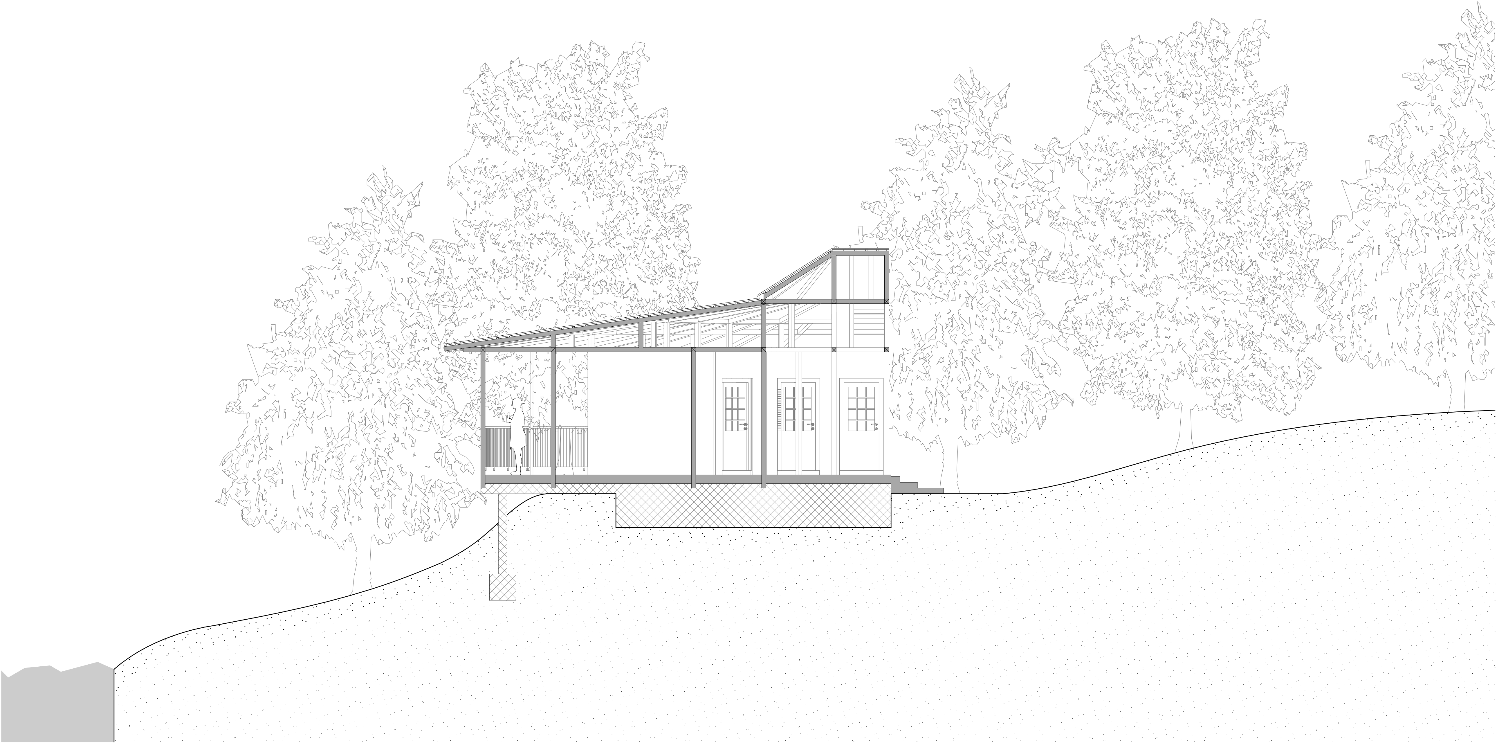
S-02 Schnitt
