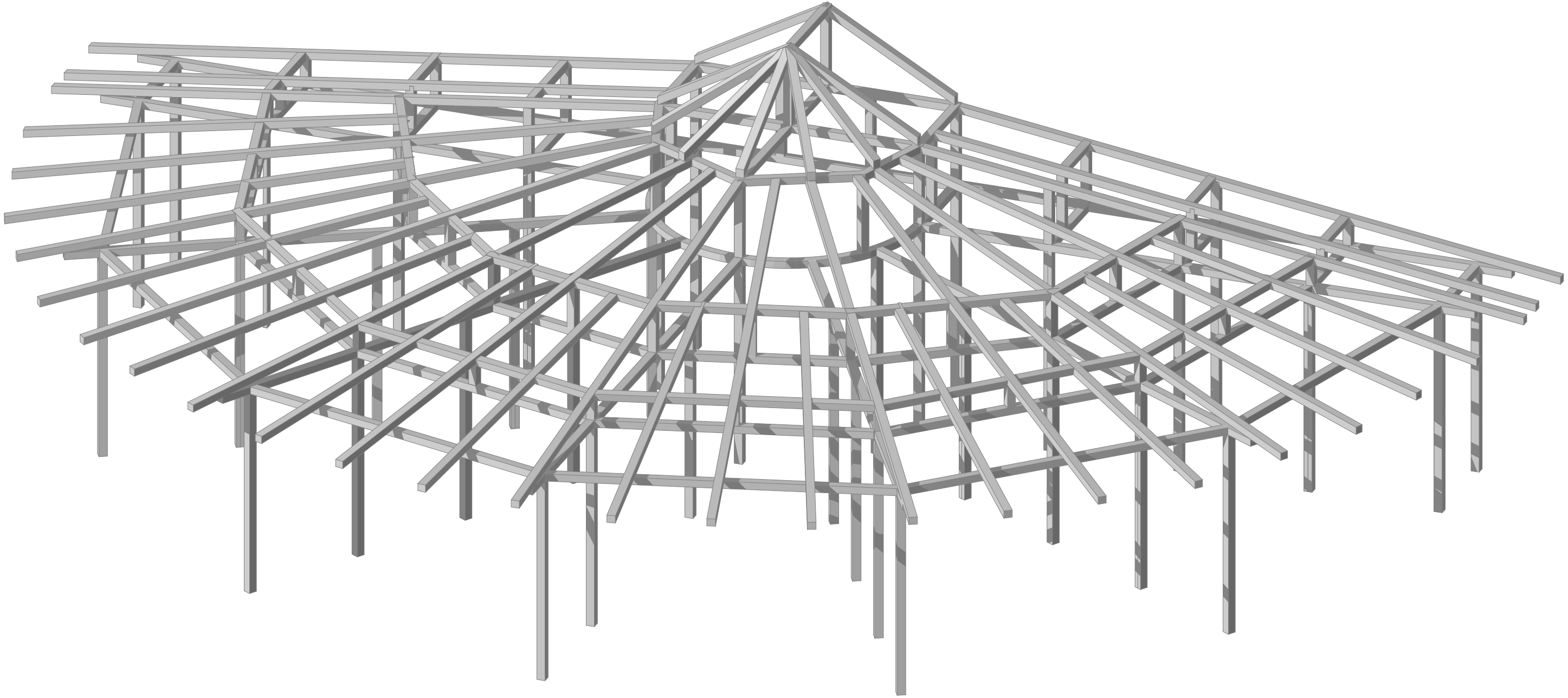
Tragkonstruktion
